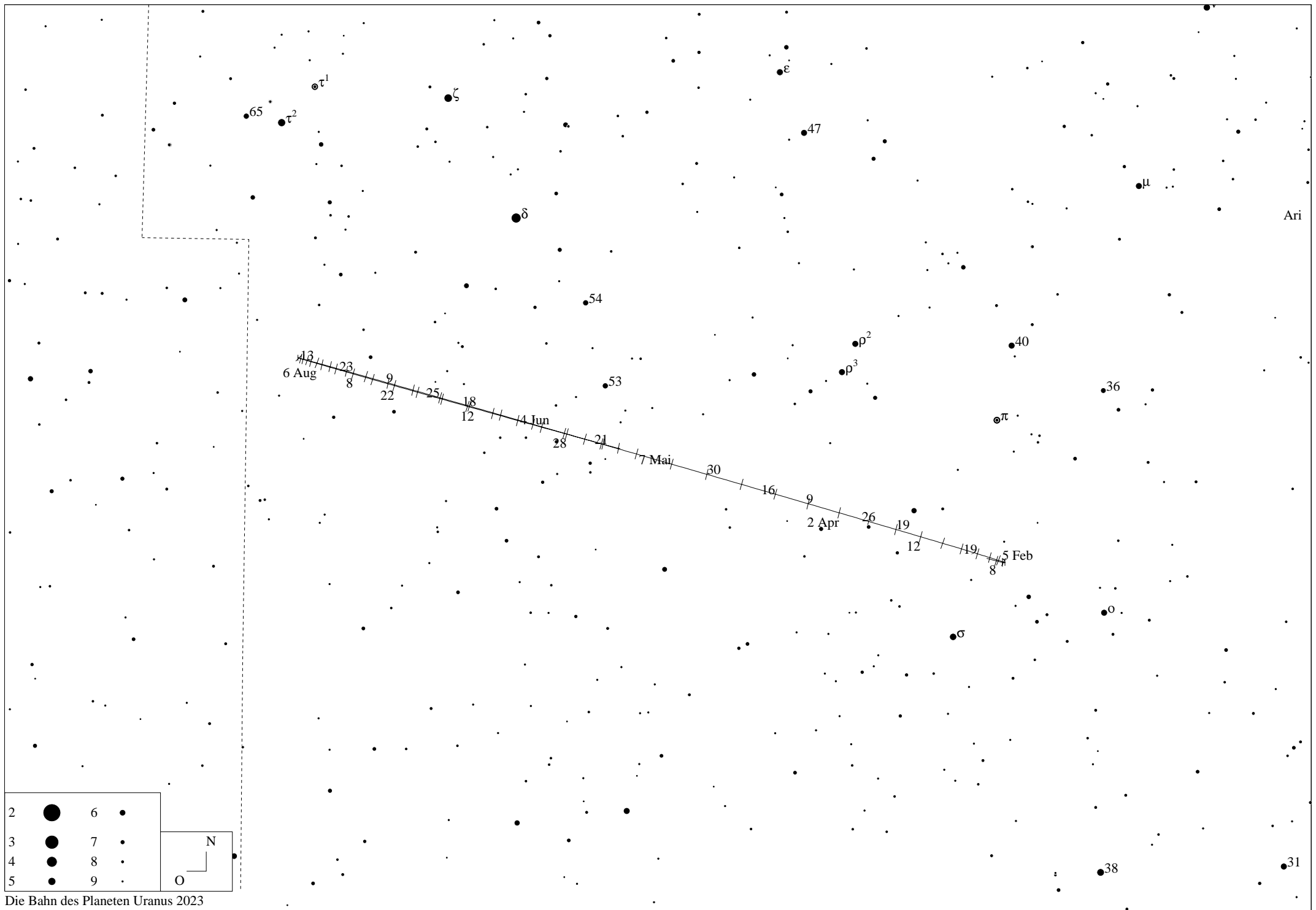
Die Bahn des Planeten Uranus 2023
