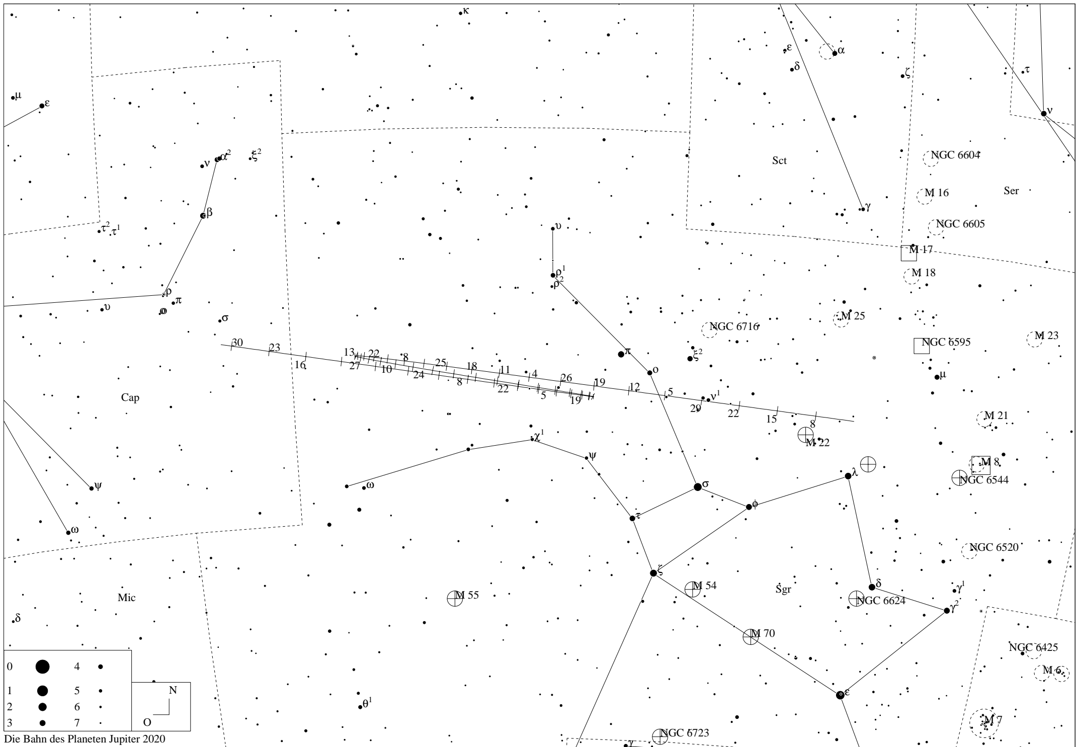
Die Bahn des Planeten Jupiter 2020
